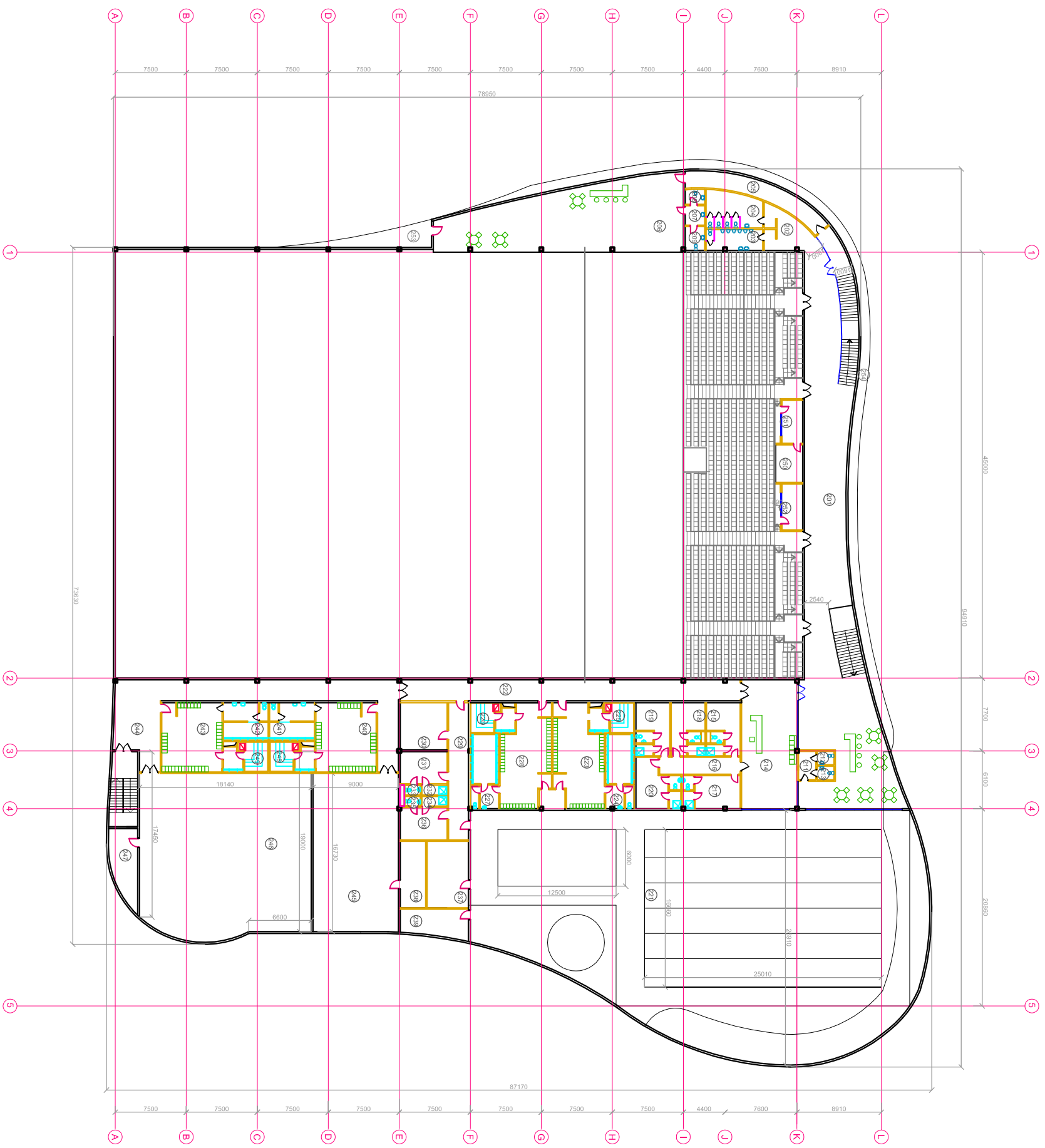
2. STĀVA PLĀNS
